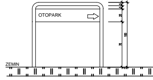
ÖN GÖRÜNÜŞ SİSTEM DETAYI Ö :1/20
