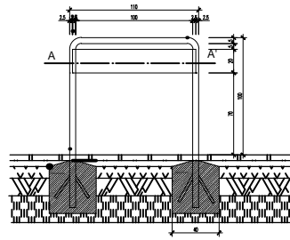
KESİT SİSTEM DETAYI Ö :1/20
