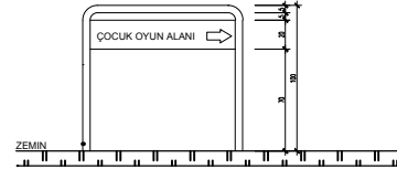
ARKA GÖRÜNÜŞ SİSTEM DETAYI Ö :1/20
