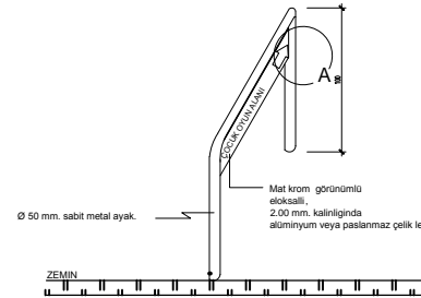
BAĞLANTI DETAYI
